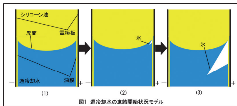
図1は、電場付与による過冷却水の凍結開始と進展状況のイメージ図である。図(1)の両端にある電極に高電圧を印加すると、図(2)中界面下部にある過冷却水が凍結を開始し、図(3)では凍結が進展している。
