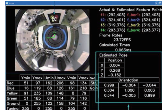
全方位カメラによる位置姿勢推定
