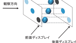
図2 輝度変調型奥行き融合錯視 (DFD) (三橋他:画像と視覚情報科学、映像情報メディア学会)
