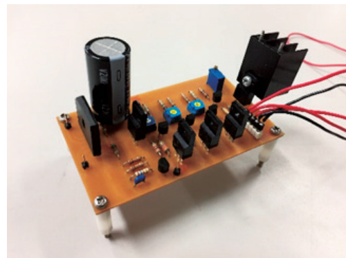
電磁波ノイズの発生しないLED駆動回路 発光効率:90%以上を実現
