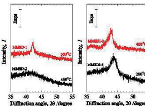
イオン照射しない場合は400℃でも結晶化しないが、イオン照射しながらTiNi成膜すると、あるイオン照射条件において200℃でも結晶化できる。
