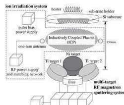
開発した多元素同時スパッタ/プラズマイオン注入成膜装置イメージ図
