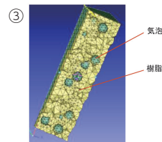
③ 発泡成形品の物性予測のための構造解析モデル
