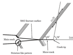
水素による破壊のモデル
