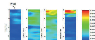
図 蒸発冷却舗装システムにおける白華進行の様子（セメント系ブロック）
