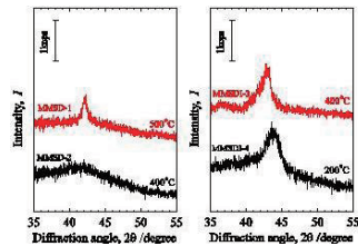
イオン照射しない場合は400℃でも結晶化しないが、イオン照射しながらTiNi成膜すると、あるイオン照射条件において200℃でも結晶化できる。
