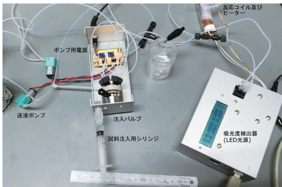
試作した簡易型流れ分析装置。送液には小指サイズのマイクロリングポンプを、反応溶液を加熱するためのヒーターにはハロゲンランプを、反応溶液の色の濃さを検出する吸光度検出器の光源にはLEDを用いています。
