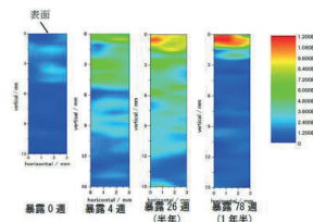
図 蒸発冷却舗装システムにおける白華進行の様子(セメント系プロック)
