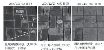
図 蒸発冷却舗装システムにおける白華進行の様子(セメント系プロック)
