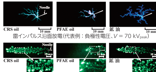
交流沿面放電(代表例：V = 35 kV rms 、電圧印加時間 30 min.)
