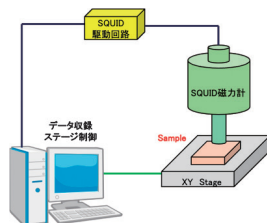
SQUID磁力計のシステム構成
