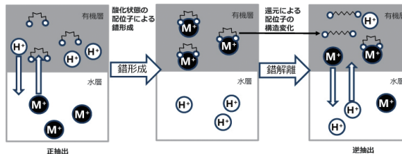
図は電氣的に特性が制御可能な配位子(抽出剤)の作用原理を示しています。配位子の分子構造変化による錯形成・錯解離を狙うものです。
