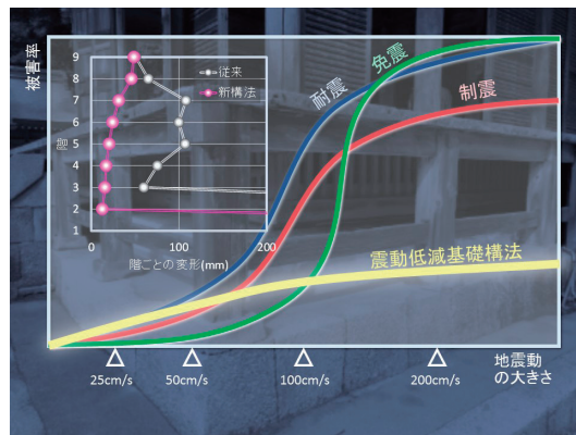
歴史的建造物の石場建てにヒントを得た震動低減基礎構法。球状砂の利用により実現することができました。
