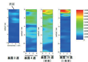
蒸発冷却舗装システムにおける白華進行の様子(セメント系プロック)
