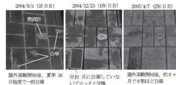
蒸発冷却舗装システムにおける白華進行の様子(セメント系プロック)
