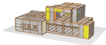
図2 解析モデル
