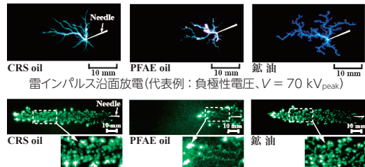
交流沿面放電(代表例: V = 35 \text{ kV}_{\text{rms}} 、電圧印加時間 30 min.)
