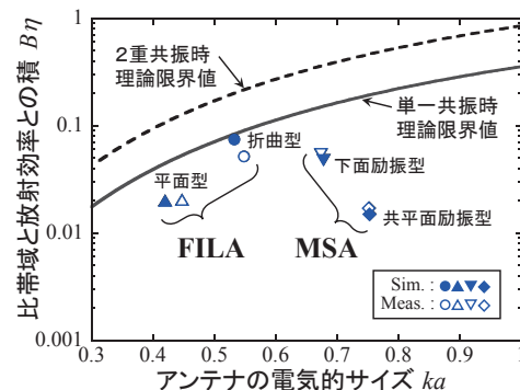
理論限界値に対する小形アンテナ(FILA, MSA)の特性例を図に表します。アンテナに折返し構造やスタブを組み込むことにより、理論限界値にせまる小型化を実現しています。
