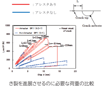
き裂を進展させるのに必要な荷重の比較
