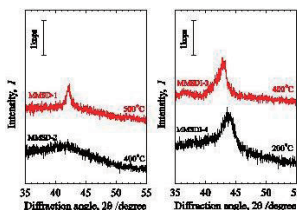
イオン照射しない場合は400℃でも結晶化しないが、イオン照射しながらTiNi成膜すると、あるイオン照射条件において200℃でも結晶化できる。
