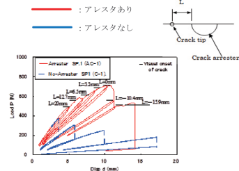
き裂を進展させるのに必要な荷重の比較
