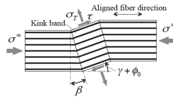
圧縮破壊のキンクバンドモデル
