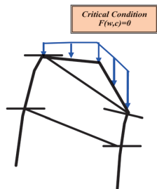
限界状態の定義と倒壊条件の導出
