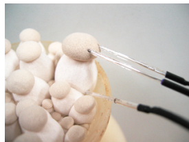
生体電位計測のためにキノコ子実体に挿入した針電極
