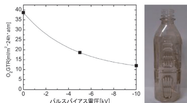
PET (厚み 100μm) の酸素ガス透過度と表面改質電圧の関係 PET (厚み 100μm) の酸素ガス透過度と表面改質電圧の関係 表面改質電圧(パルスバイアス電圧)を高くすることで、酸素ガス透過度をより低くすることができる。ガラスの値(ほぼ0)を目標としてさらなる改善に取り組んでいる。
