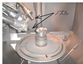
図2. 微粒子処理装置の例
