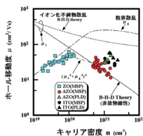
ZnO系透明導電膜の電気伝導機構
