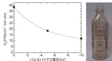
PET(厚み100μm)の酸素ガス透過度と表面改質電圧の関係 表面改質電圧(パルスバイアス電圧)を高くすることで、酸素ガス透過度をより低くすることができる。ガラスの値(ほぼ0)を目標としてさらなる改善に取り組んでいる。
